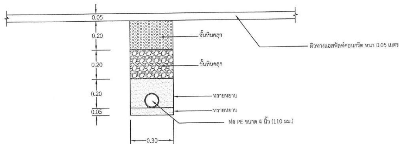
แบบขยายชุดวางท่อผ่านถนนลาดยาง
