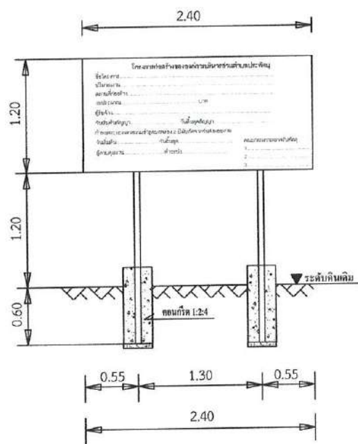
รูปด้านหน้า NOT TO SCALE
