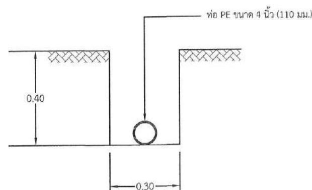
แบบขยายจุดวางท่อ มาตราส่วน NOT TO SCALE
