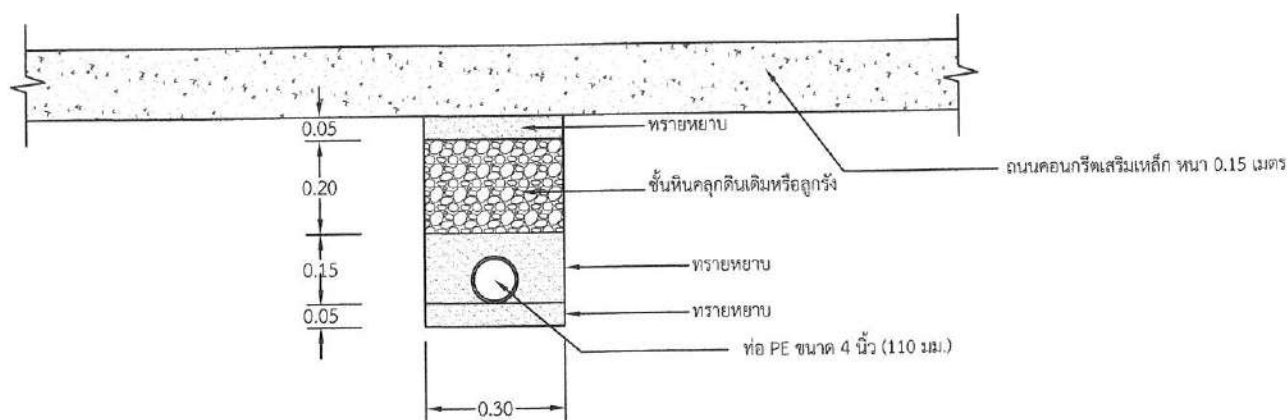
แบบขยายชุดวางท่อผ่านถนนคอนกรีต
