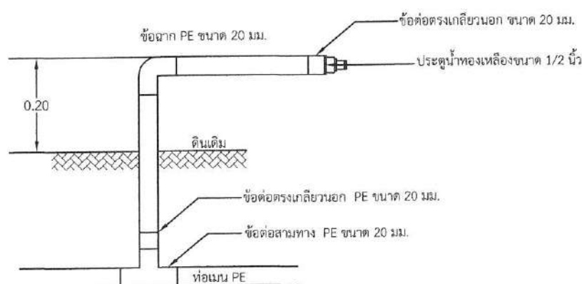
แบบการติดตั้งจุดจ่ายน้ำ มาตราส่วน NOT TO SCALE
