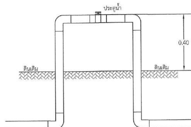
แบบการติดตั้งประตุน้ำ มาตราส่วน NOT TO SCALE
