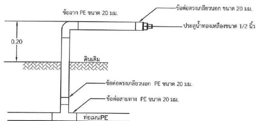
แบบการติดตั้งจุดจ่ายน้ำเข้าบ้าน ขนาดส่วน NOT TO SCALE
