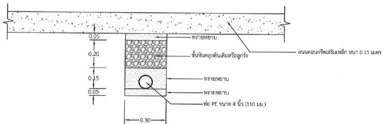
แบบขยายชุดวางท่อผ่านถนนคอนกรีต มาตราส่วน NOT TO SCALE
