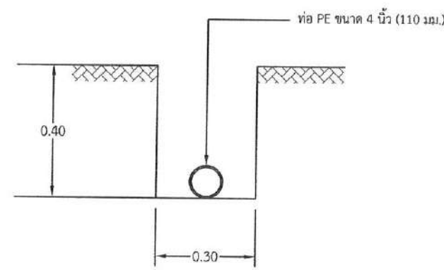
แบบขยายชุดวางท่อ ขนาดส่วน NOT TO SCALE
