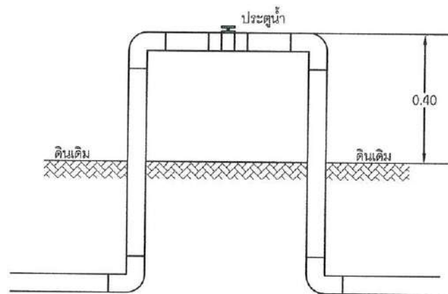
แบบการติดตั้งประตุน้ำ ขนาดส่วน NOT TO SCALE
