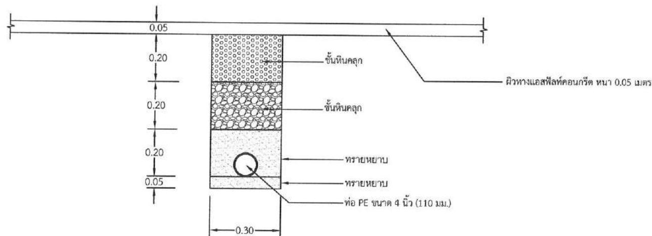
แบบขยายชุดวางท่อผ่านถนนลาดยาง มาตราส่วน NOT TO SCALE
