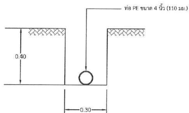
แบบขยายชุดวางท่อ มาตราส่วน NOT TO SCALE
