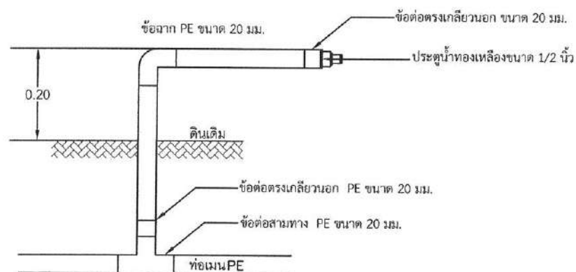
แบบการติดตั้งจุดจ่ายน้ำเข้าบ้าน มาตราส่วน NOT TO SCALE
