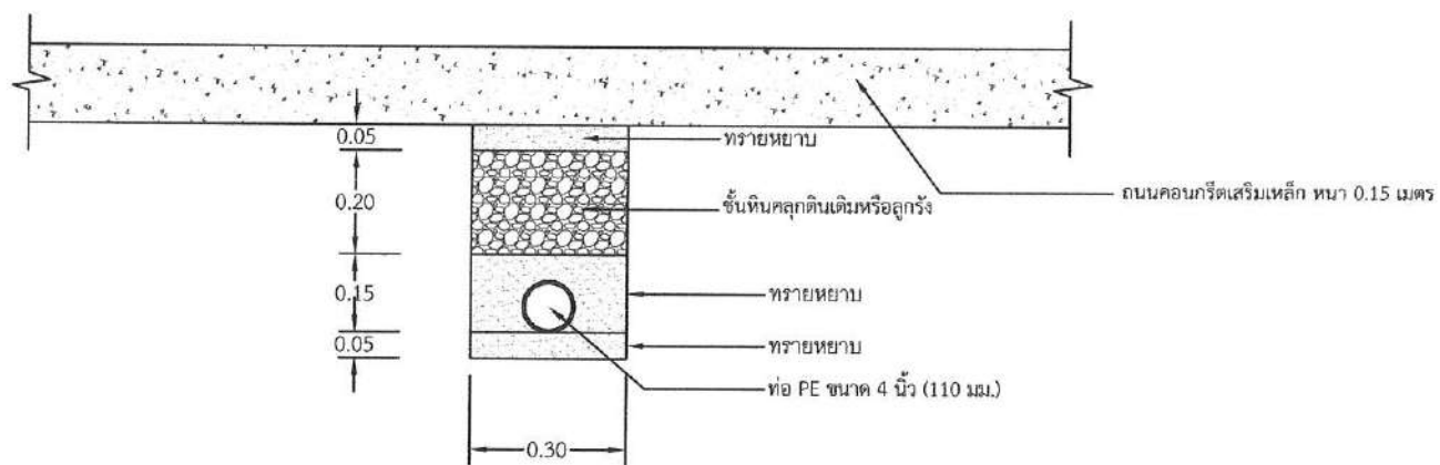
แบบขยายชุดวางท่อผ่านถนนคอนกรีต
